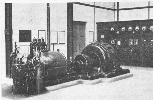
Bild 8. Kraftzentrale
