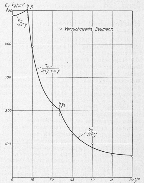
Bild 3. Druckfestigkeit der Gotthardtanne
