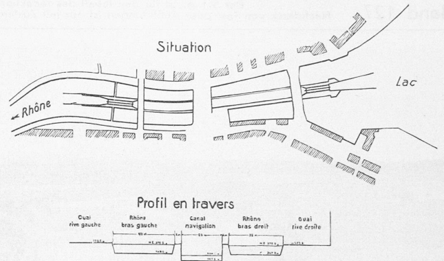
Bild 6. Vertiefte Mittelrinne für die Schifffahrt in der Rhone: In der obren Schleuse würden die Schiffe so tief abgesenkt, dass sie unter den Brücken hindurch kommen, in der untern würden sie wieder auf Höhe des Rhonespiegels gehoben
