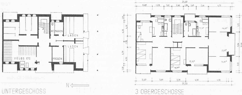
UNTERGESCHOSS OBERGESCHOSS Grundrisse der fünfgeschossigen Blöcke B mit Zwei- und Dreizimmerwohnungen
