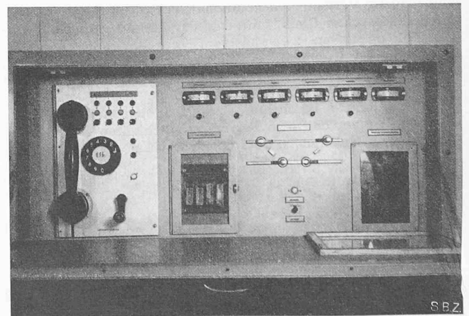
Bild 5. Kontrolltafel der ferngesteuerten Signalstation in Tunnelmitte mit Bedienungsstand für die lokale Betätigung der Weichen
