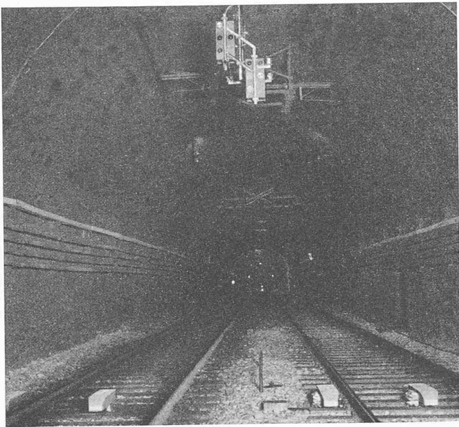
Bild 4. Einfahrtsignal mit Ausfahrsvorsignal der Signalstation Gotthard. Beide Gleise sind für automatische Zugbeeinflussung ausgerüstet (wegen wahlweise eingleisigem Betrieb)
