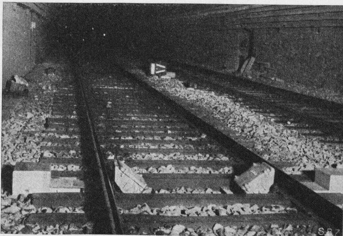
Bild 6. Induktive Impulsgeber für die Achszählung
