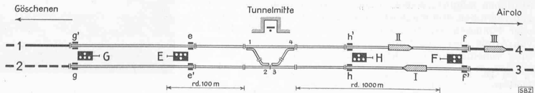
Bild 3. Lageplan der Signalstation in Tunnelmitte
