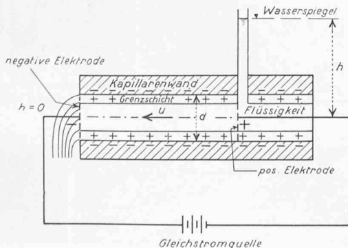
Bild 4. Schema der hydraulisch-elektrosmotischen Kapillarströmung
