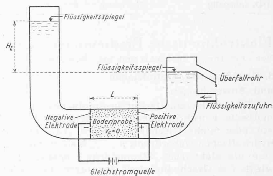
Bild 7. Schema der elektromotischen Steighöhenmessung
