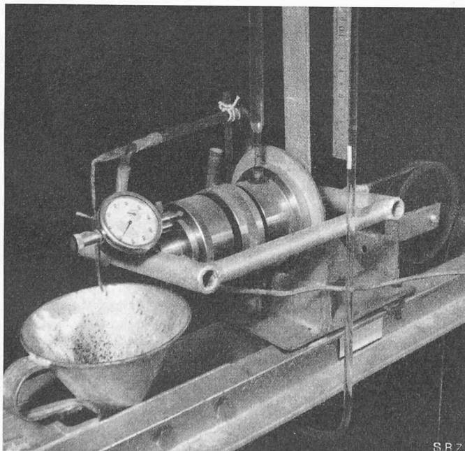
Bild 9. Für Steighöhenversuche umgebautes normales Oedometer mit Steigrohr (rechts) und kommunizierendem Gasentlüftungrohr (links)
