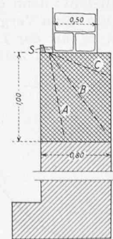
Bild 14. Unterfangung des Gebäudes für das Kolonialministerium, Paris
