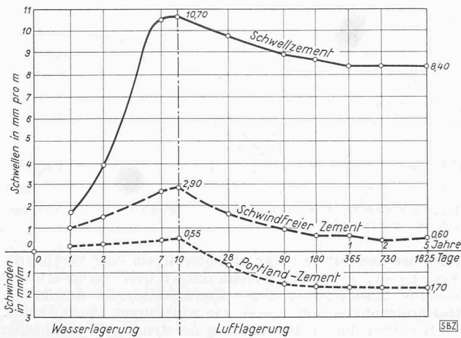
Bild 7. Schwellen und Schwinden verschiedener Zemente bei zehntägiger Wasser- und anschließender Luftlagerung
