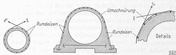
Bild 2. Rohre mit vorgespannter Umschnürung nach Emperger, 1923
