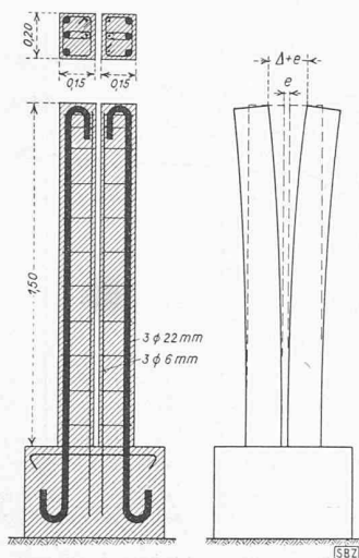
Bild 10. Zwei Versuchsprismen auf gemeinsamem Fundament, links frisch betoniert, rechts später
