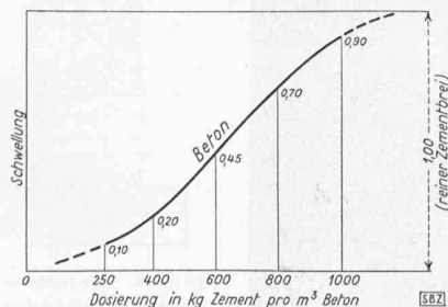
Bild 8. Relative Schwellung von Beton in Funktion seiner Dosierung
