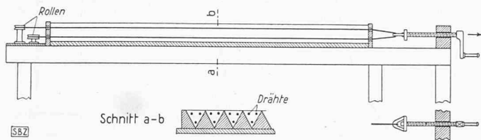
Bild 1. Herstellung von Spannbeton nach Doehring, 1888
