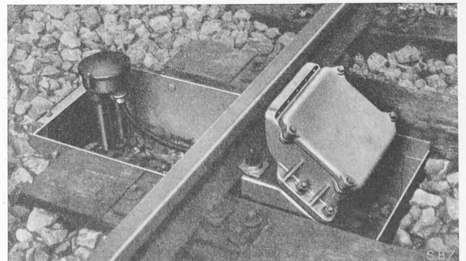
Bild 4. Induktiver Impulsgeber für den automatischen Streckenblock mit Achszählung
