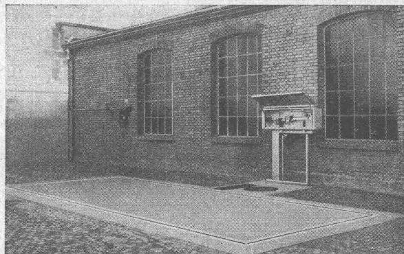
Brückenwaage für Strassenfahrzeuge, Wiegefähigkeit 20 t. Mit Betonbrücke, torsionsfreiem Hebelwerk und verstellbaren Schneiden
