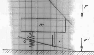
Bild 1. Schematische Darstellung einer Anordnung zur Körperschalldämmung.
