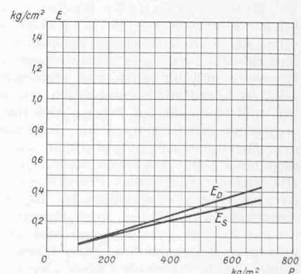
Bild 9. Glasseidematte, 2 kg/m 2
