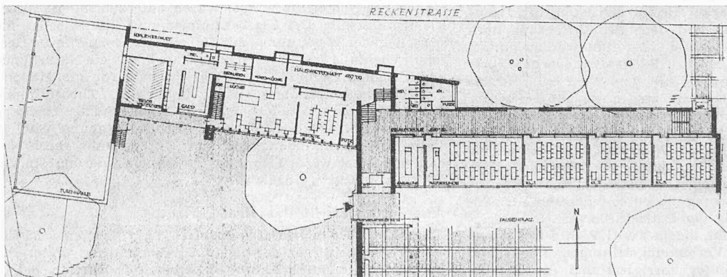
Erdgeschoss 1 : 700
