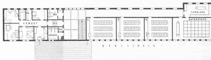
Obergeschoss 1:700
