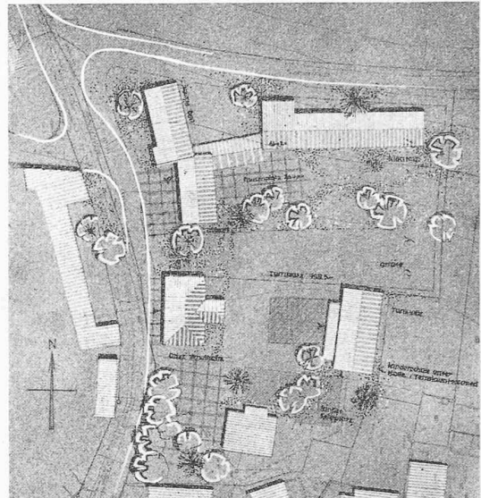
Lageplan 1 : 2000
