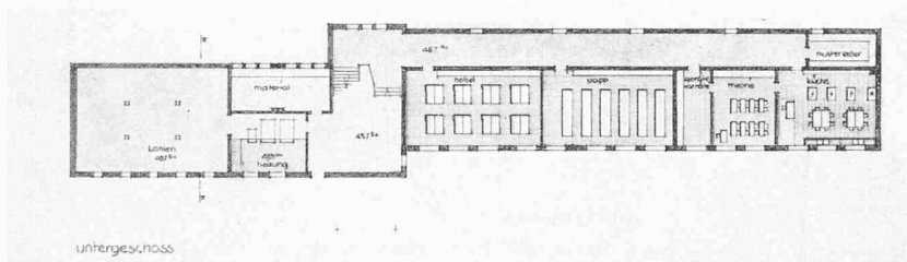
Untergeschoss 1 : 700
