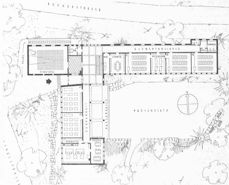
Erdgeschoss 1:700
