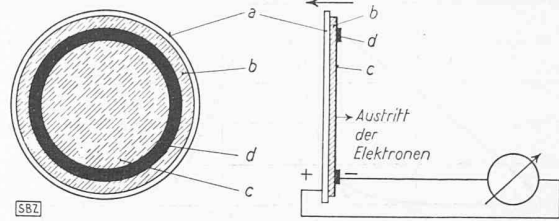
Bild 1. Selenphotoelement. a Eisenscheibe, b Selenschicht, c Edelmetallhaut, wirkt als Vorderelektrode, d Metallring zur Stromzuführung
