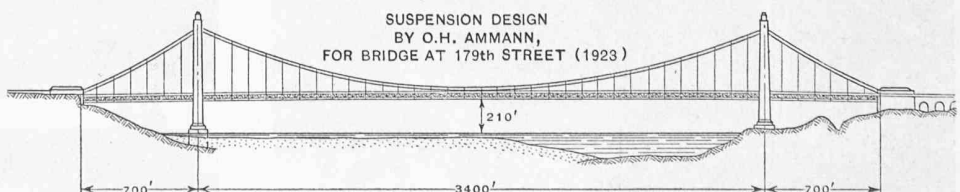
Bild 26. Jüngere Entwürfe für Brücken über den Hudson River in New York, zu unterst der ausgeführte Entwurf der George Washington Bridge von O. H. Ammann. 1 : 135 000
