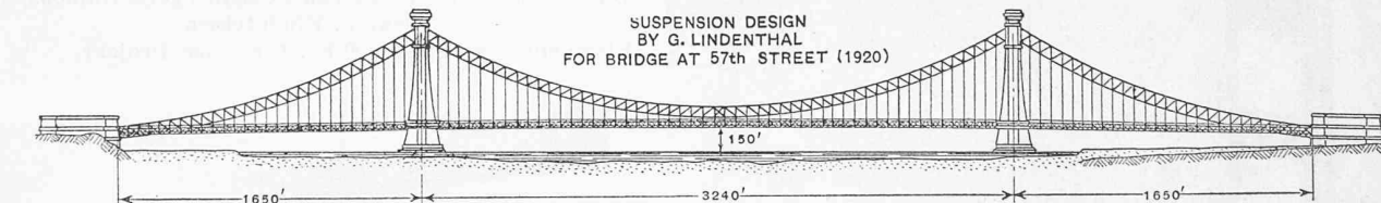
Bild 25. Aeltere Entwürfe für Brücken über den Hudson River, 1 : 135 000
