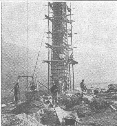
Schalung eines Betonmastes
