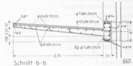
Bilder 8 und 9. Schnitte des Vordaches an der Eisenbetondecke Bild 7, Masstab 1 : 70. Ing. A. WICKART, Zürich
