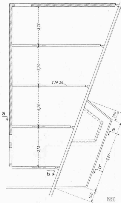
Bild 7. Kopfbau, Decke über dem eingeschossigen Teil, 1 : 200
