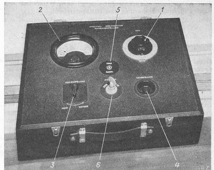
Bild 19. Tragbarer Steuerkasten für den Gebläseantrieb. 1 Drehzahlinsteller, 2 Stellungsfernanzeiger der Feineinstellung, 3 Feineinsteller «Mehr — 0 — Weniger», 4 Notknopf, 5 Umschalter «Hand» — «automatisch», 6 Sicherheitsschlüssel
