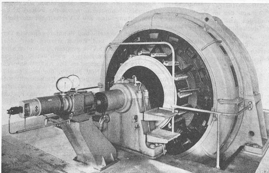
Bild 25. Betriebsmotor des grossen Gebläses mit angebaubtem Reguliergetriebe, Kontrolltachometern und Steuerfrequenzgenerator
