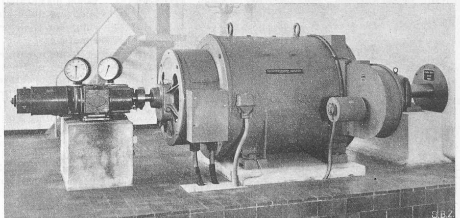
Bild 23. Antriebsmotor des kleinen Gebläses mit angebautes Ventilator zur Fremdbelüftung (rechts) und Reguliergetriebe mit Steuerfrequenzgenerator (links)
