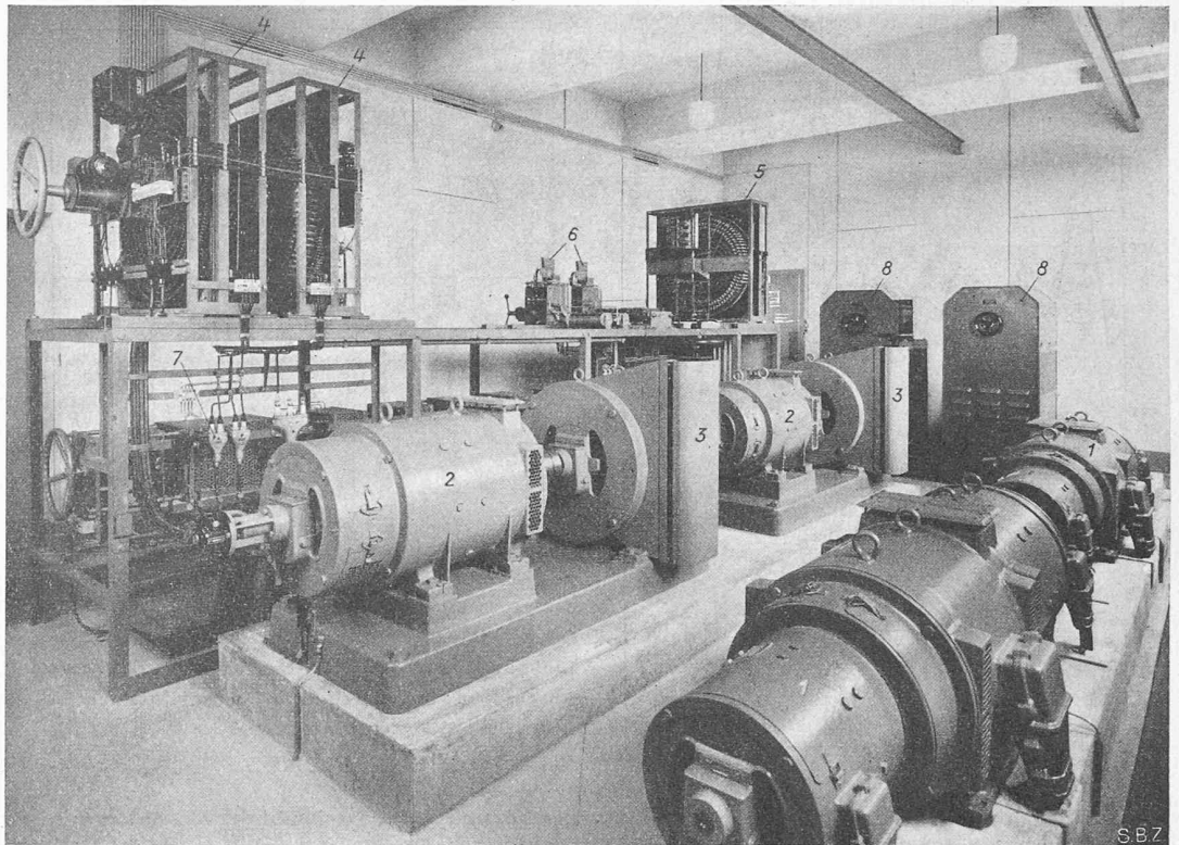
Bild 22. Regulier- und Hilfsaggregate. 1 Einwellen-Umformer Drehstrom-Gleichstrom, 2 Mittelfrequenz-Generatoren mit Gleichstromantrieb, 3 Wicklungsumschalter, 4 Hauptpotentiometer für den Antrieb des grossen Gebläses, 5 wie 4 für das kleine Gebläse, 6 Entregungsschalter, 7 Regulierapparate der Propellermotoren, 8 Oeldruck-Steuerfrequenzregler der beiden Gebläseantriebe
