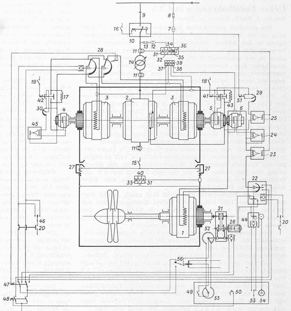
Bild 18. Prinzipschema des elektrischen Antriebes für das Gebläse des grossen Windkanals.
