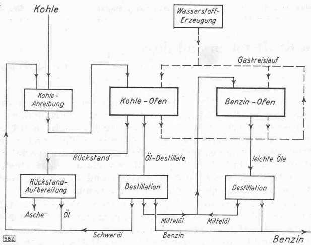
Bild 2. Schema der Benzingewinnung aus Kohle
