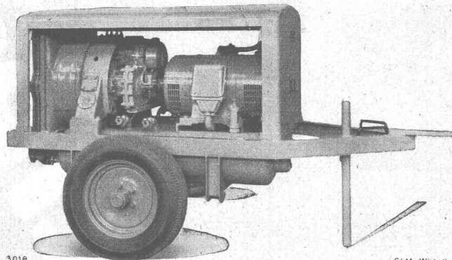
3016 Zweiradaggregat mit Luftkühlung und Elektromotorantrieb, 4,6 m 3 /min. eff. SLM-Winterthur
