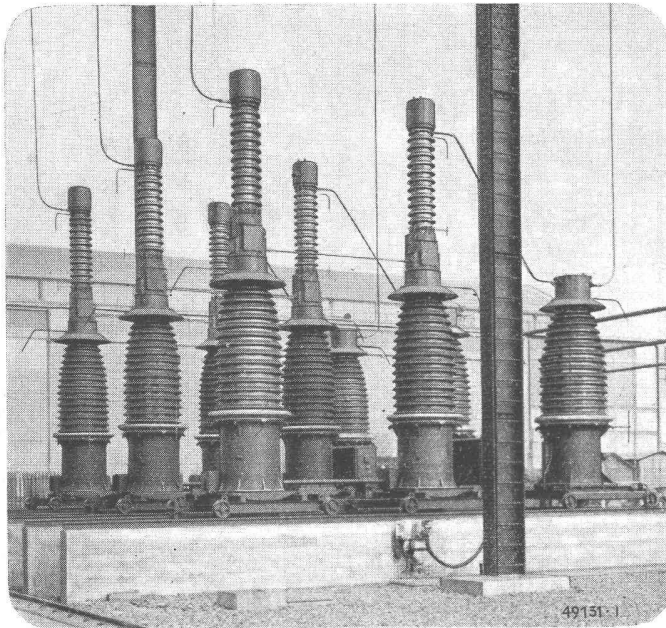
Oelarmer Hochspannungs-Schnellschalter für 230 000 Volt Betriebsspannung und 3 500 000 kVA Ausschaltleistung
