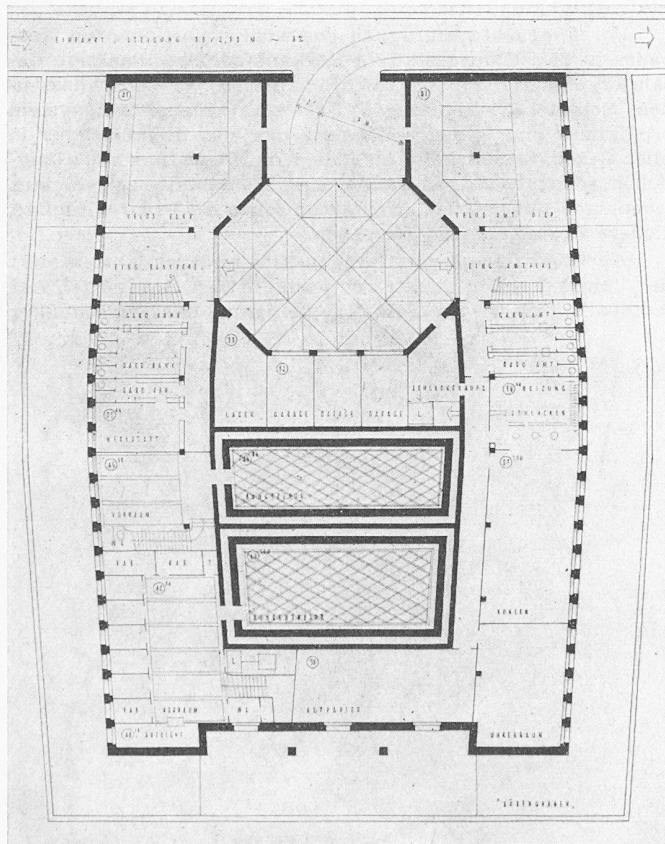
Untergeschoss 1:600
