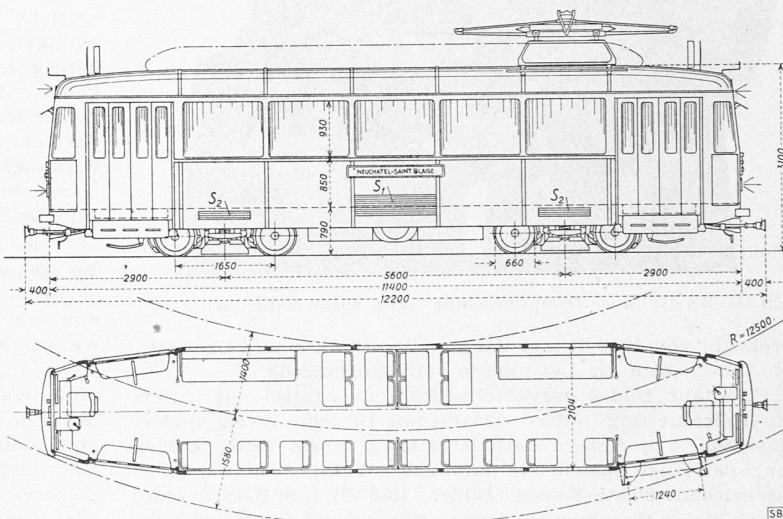
Bild 2. Typenskizze, Masstab 1 : 120
