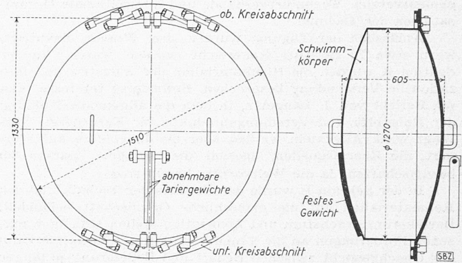
Bild 8. Abschlussdeckel, Masstab 1:30
