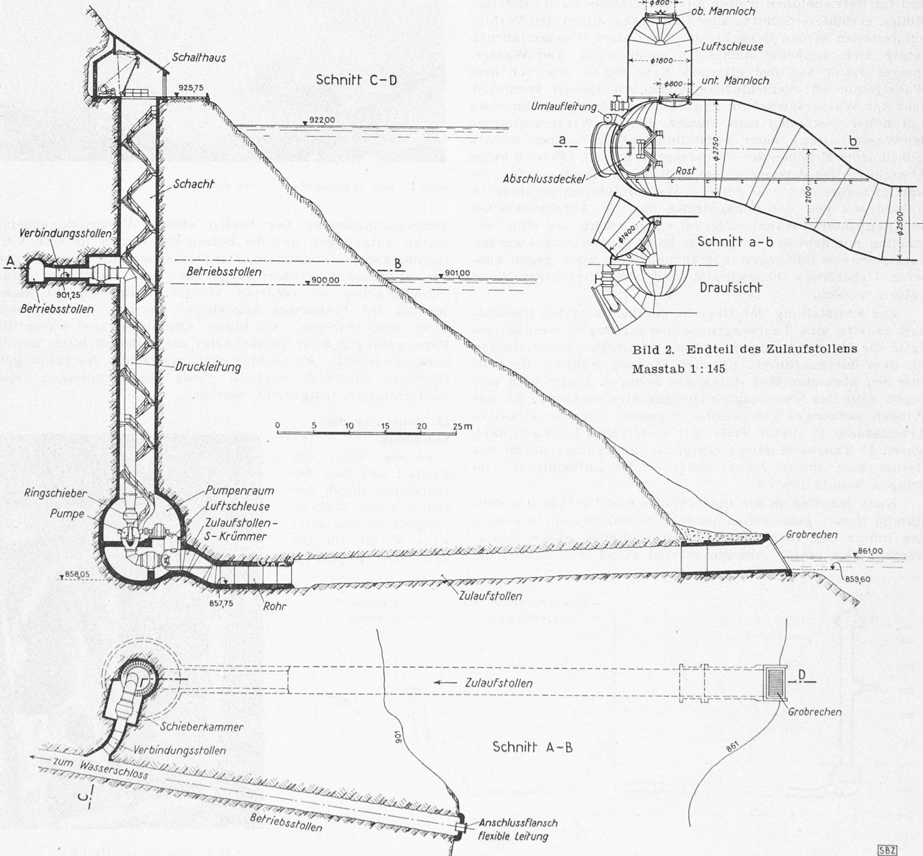
Bild 1. Schachtpumpenanlage mit neuer Wasserfassung im Vorderen Gosausee, Salzkammergut. Masstab 1 : 700
