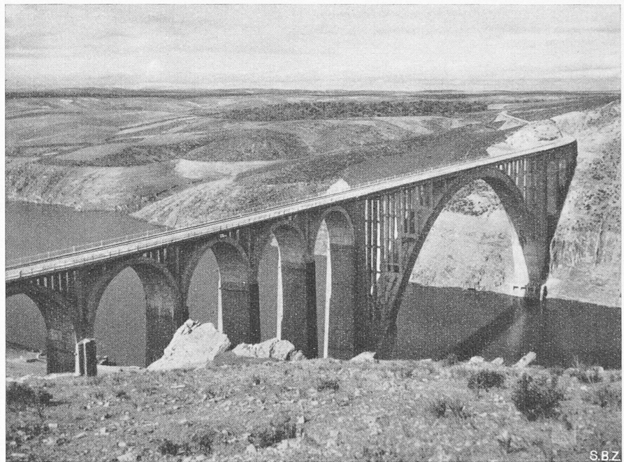
Bild 2. Martin Gil-Viadukt über den Esla-Fluss
