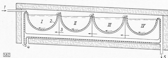
Bild 1. I bis IV Gefrieraschen, 1 Saft Eintritt, 2 Siebband, 3 Soledurchtritt von einer Tasche zur andern, 4 zur Zentrifuge, 5 Konzentrat-Austritt
