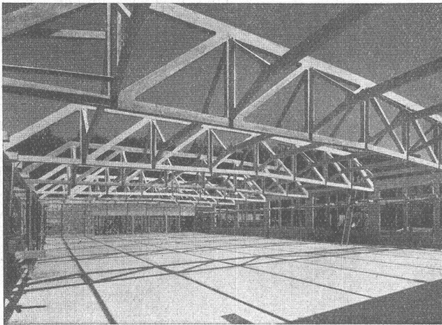
Eisenbetonfachwerk - Montagefertig
