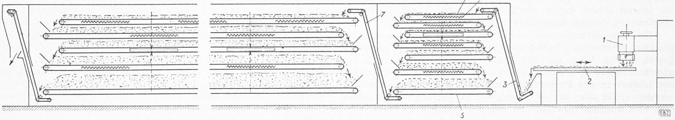
Bild 8. Prinzipschema eines Bandrockners für Kurzwaren. 1 Teigwarenpresse, 2 Schüttelsieb, 3 Elevator, 4 oberes Transportband, 5 unteres Transportband, 6 Lufterhitzer, 7 Elevator
