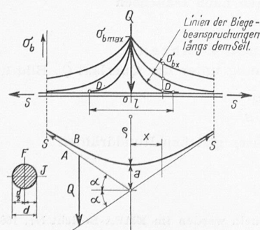
Bild 1. Schematische Darstellung der Biegelinien und Linien der Biegebeanspruchungen an Stahlseilen mit verschiedenem Steifigkeitsgrad
