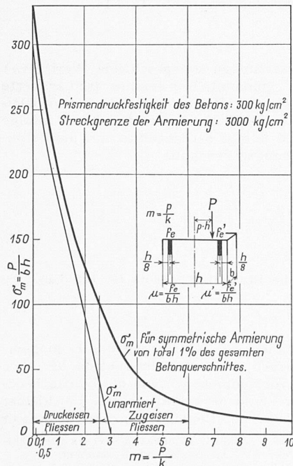
Bild 2. Exzentrischer Druck
