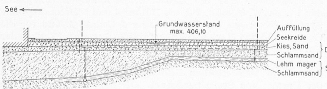
Bild 10. Numerierung der sechs Häuser, Dilatationsfugen D (zwischen Haus 2 u. 3 keine); Rammsondierungen R, Bohrungen B und Schächte S; geologisches Profil. Masstab 1:1750
