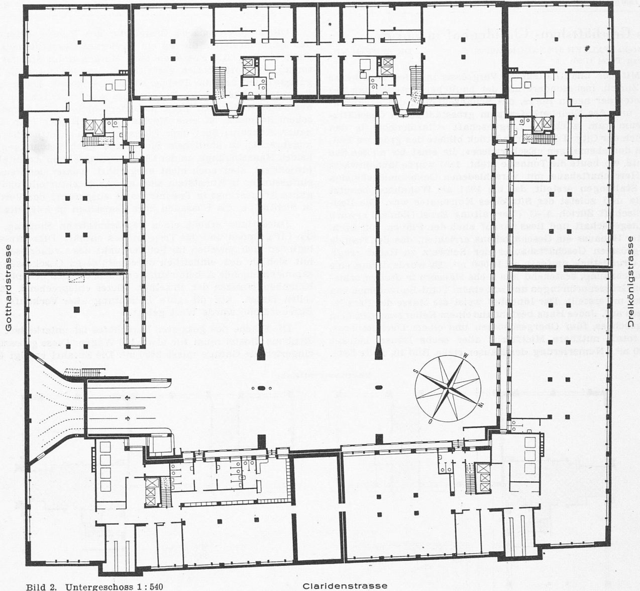
Bild 2. Untergeschoss 1 : 540
