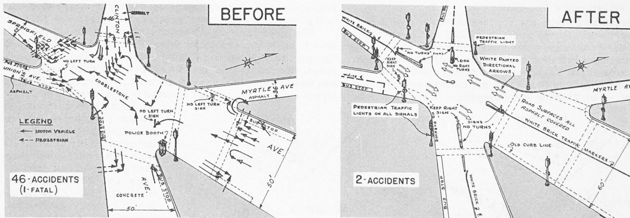
Bild 5. Problem: In der vierjährigen Periode von 1935 bis 1939 gab es auf dieser Kreuzung von drei Strassen in Irvington, N. J., 46 Unfälle mit 30 Körperverletzungen und einem Todesfall; in diese Unfälle waren 22 Fussgänger verwickelt. Der Gesamtschaden betrug 17 400 $. Verkehrsstudien: Das Dreiphasensignal erwies sich als unzweckmässig eingestellt, da es verkehrshemmend wirkte und zu Zusammenstössen führen konnte. Die Verkehrszählungen ergaben ein Mittel von 27 700 Fahrzeugen und 40 000 Fussgängern während 14 Stunden von Wochentagen, von 7.00 bis 21.00 Uhr.
