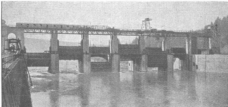
Kraftwerk Eglisau
