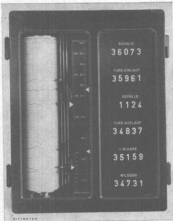
Kraftwerk Ruppertswil-Auenstein Registrierende Wasserstandsfernmelder für 5 Wasserstände und das Neftogefälle
