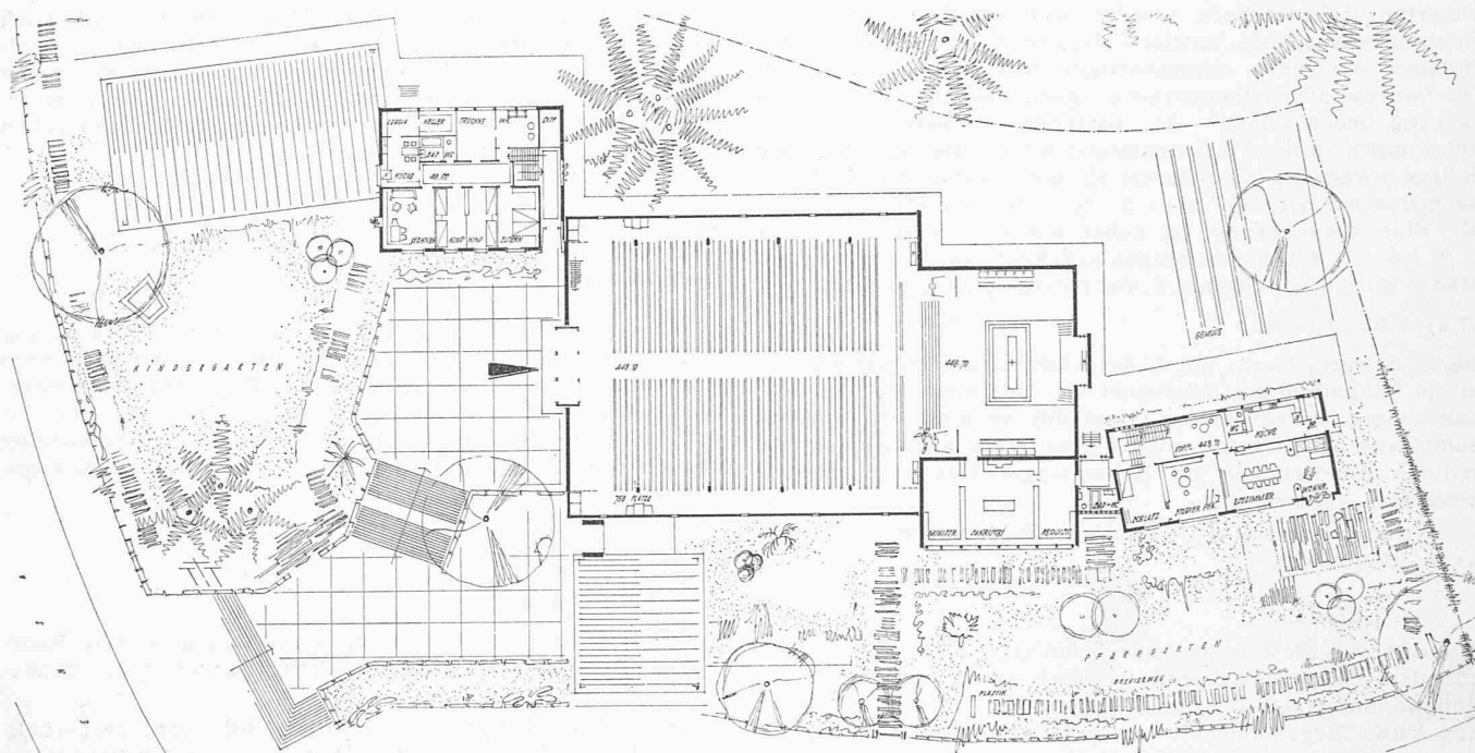
Erdgeschoss 1:600
