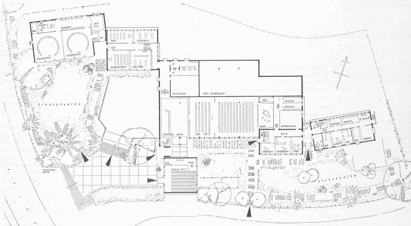
Untergeschoss 1:600
