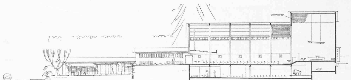
1. Preis. Längsschnitt 1: 600
