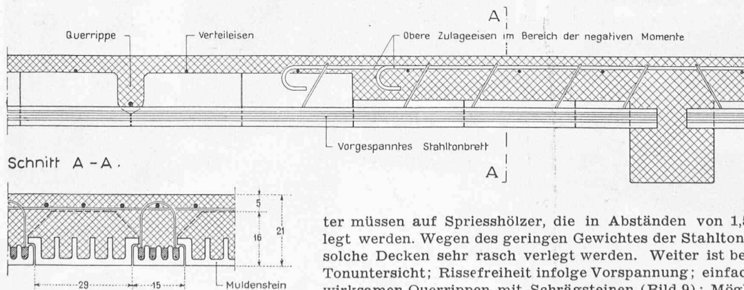
Bild 9. Kontinuierliche Stahltondecke, 1:15
