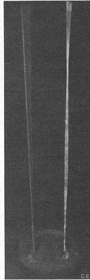
Bild 11. Um 45^\circ verwundener Stab 40/4. Oberer Knotenpunkt in Abstand 0,284 der Schaufellänge von der Spitze
