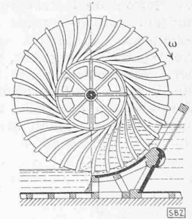
Bild 10. Zuppinger-Wasserrad
