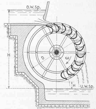
Bild 4. Oberschlächt. Wasserrad
