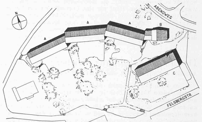
Bild 2. Lageplan, Masstab 1 : 2000. A Klassenpavillon, B Singsaal, C Turnhalle
