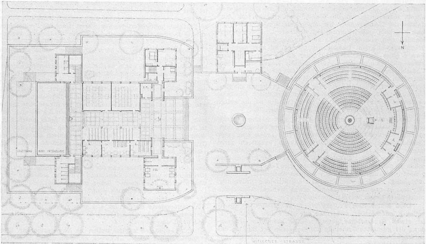
Grundriss 1:600
