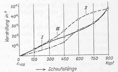
Bild 28. Abhängigkeit der Verdrillung von der Entfernung vom Schauffuss für drei in der Breite verjüngte Schauffeln von gleichbleibender Dicke 16 mm. Verjüngung:
