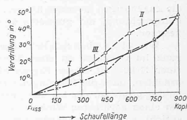
Bild 28. Abhängigkeit der Verdrillung von der Entfernung vom Schauelfuss für drei in der Breite verjüngte Schaukeln von gleichbleibender Dicke 16 mm. Verjüngung: Schaufel I 8,2/3, Schaufel II 8,2/5,7, Schaufel III 8,2/3,8
