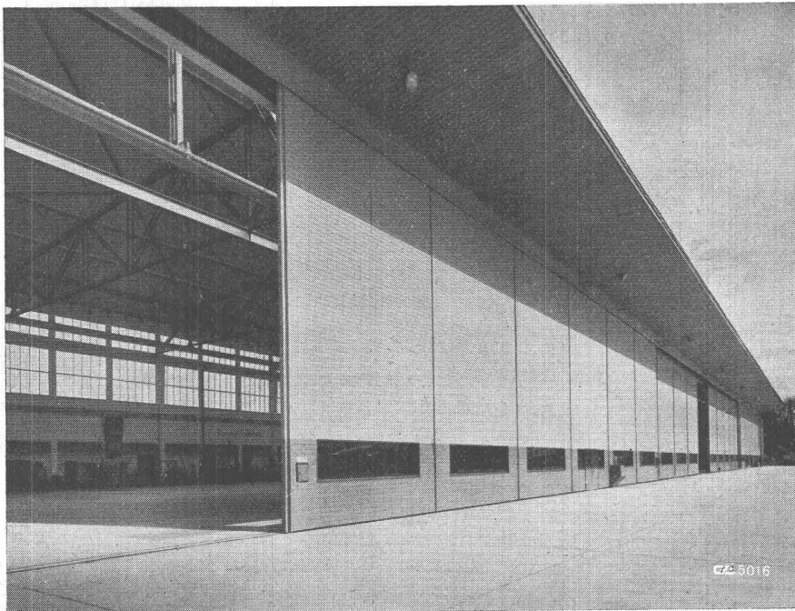
Schiebetor Werfthalle Kloten
