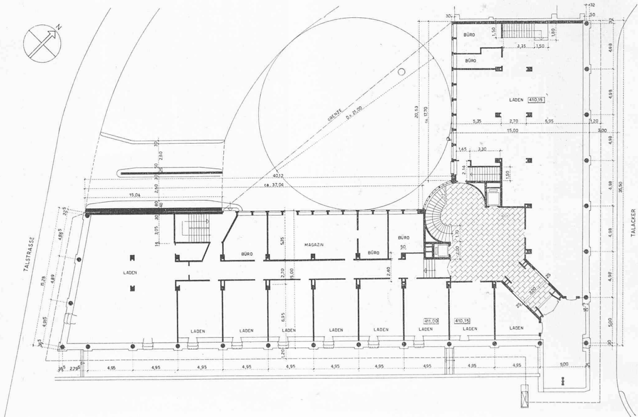
Bild 11. Erdgeschossgrundriss 1:400
