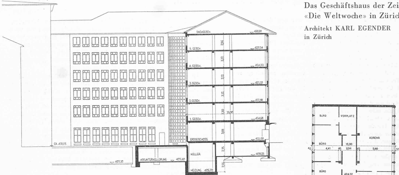
Bild 9. Schnitt 1:400
