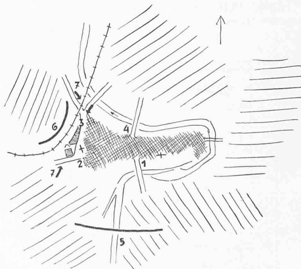
Bild 1. Radialverbindungen und Umfahrungslinien. 1 Kirchenfeldbrücke, 2 Bubenbergplatz, 3 Bollwerk, 4 Kornhausbrücke. Die Umfahrungslinien: 5 projekt. Aarebrücke, 6 Grosse Schanze oder weiter nördlich, 7 Strassentunnel, eine Fehldisposition
