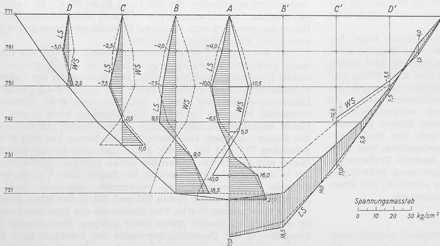
Bild 10. Verlauf der vertikalen Normalspannungen, LS = Luftseite, WS = Wasserseite
