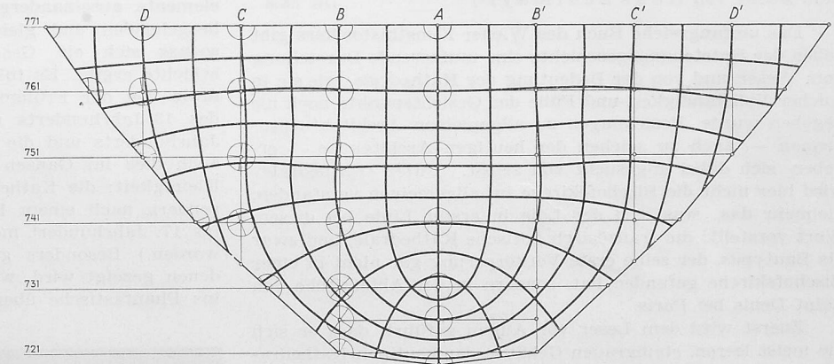
Bild 13. Hauptspannungstrajektorien an der Luftseite
