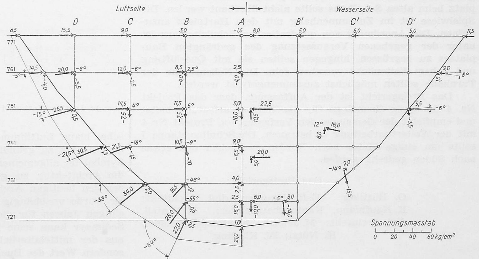
Bild 12. Hauptnormalspannungen
