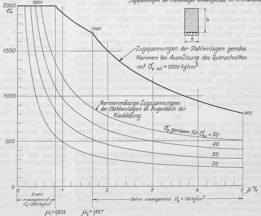
Bild 3. Rechteckquerschnitt. Rechnerische Zugspannungen der Stahleinlagen unmittelbar nach Rissbildung (Querschnitt gerissen). Vergleich mit den Zugspannungen bei Ausnützung des Querschnittes
