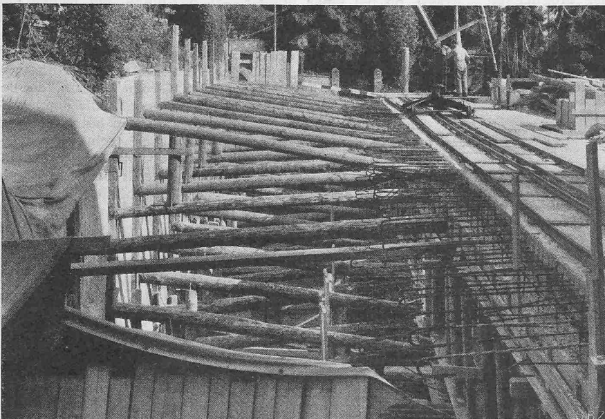
Bild 10. Spriessung für die letzte Bauetappe. Bauunternehmung Brunner & Co., Zürich
