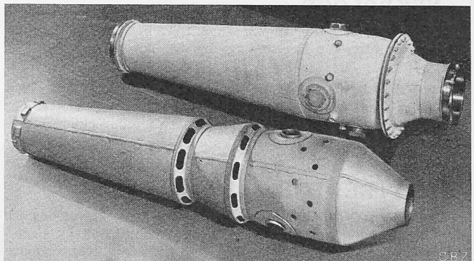
Bild 8. Brennkammer zur Turbine Bristol «Proteus»
