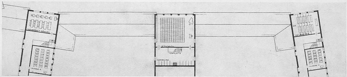
Obergeschossgrundriss 1 : 800
