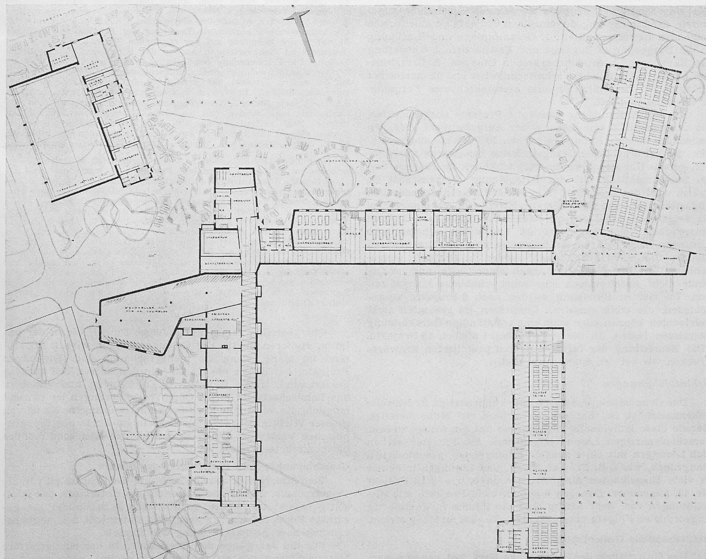
Grundriss Untergeschoss 1:800
