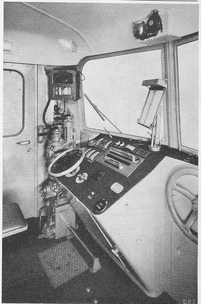
Bild 19. Führerstand der C 0 C 0 -Lokomotive
