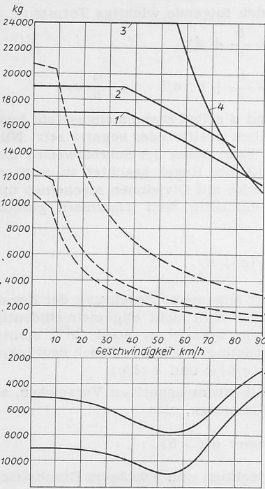
Bild 13 (links). Einphasen-Lokomotive für 20 kV, 50 Hz, Zugkräfte bzw. Bremskräfte in Abhängigkeit der Geschwindigkeit 1 Dauerzugkraft 2 Einstundenzugkraft 3 Maximale Zugkraft 4 Zugkraft auf letzter Stufe 5 Einstundenbremskraft 6 Maximale Bremskraft Gestrichelt: Zugkräfte im Gleichstrombetrieb 1500 V: 7 Dauerzugkraft 8 Einstundenzugkraft 9 Maximale Zugkraft
