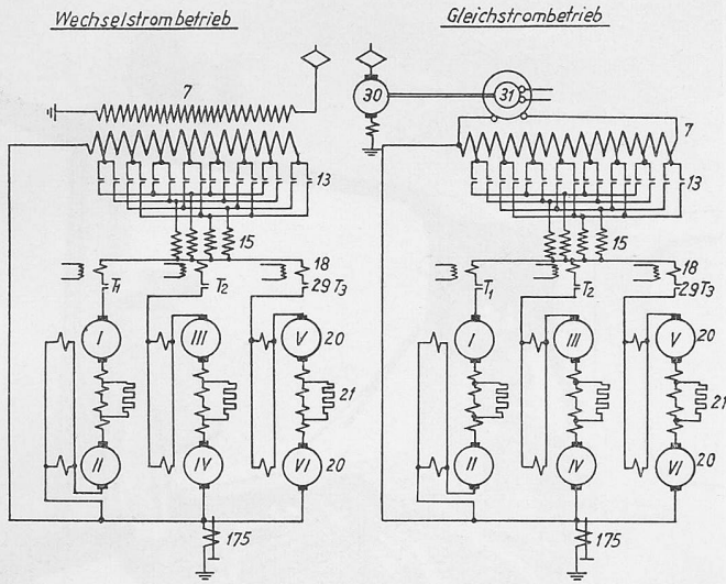
Bild 16. Hauptstromschema für die drei Betriebsarten.
