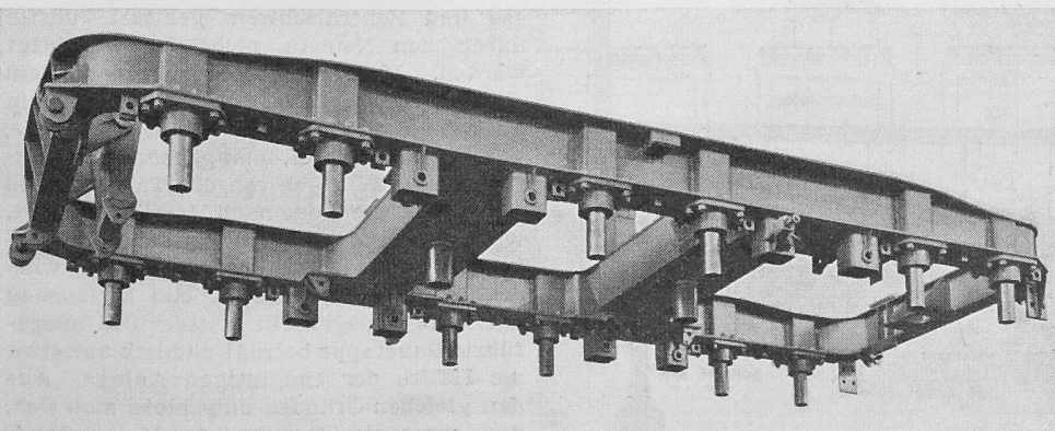
Bild 23. Drehgestellrahmen
