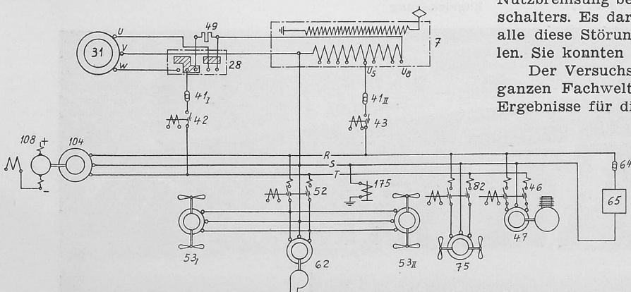
Bild 17. Schema der Hilfsbetriebe. 7 Haupttransformator, 28 Regimeschalter, 31 Wechselstromgenerator, ein- und dreiphasig, 41I und 41II Sicherungen für das Hilfsbetriebsnetz, 42 Hilfshüpf Phase T, 43 Hilfshüpf Phase R, 46 Hüpf zu 47, 47 Motor zum Bremskompressor, 49 Anlasswiderstand, 52 Hüpf zu 62, 53I und 53II Kühlluftventilatoren für die Triebmotoren, 62 Motor zur Transformator-Ölpumpe, 64 Sicherung zu 65, 65 Führerstandheizung 380 V, 75 Kühlluftventilatoren für die Triebmotor-Shunts, 82 Hüpf zu 75, 104 Arnoumformer, 108 Ladegenerator, 175 Erdschlussrelais
