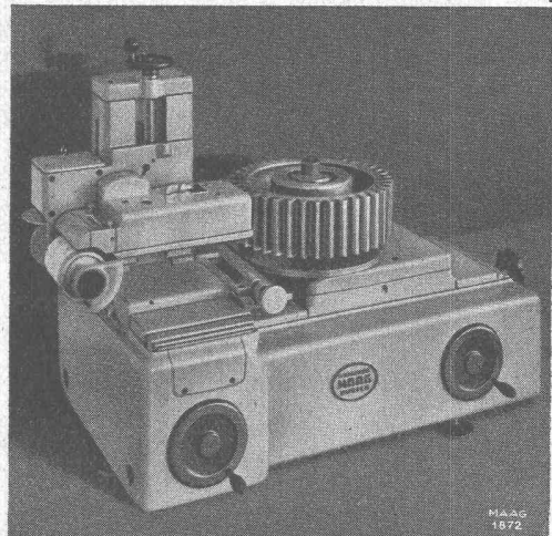
Zahnschrägemessgerät, Typ HM-30, für Stirn- und Schraubenträger bis 300 mm Durchmesser.
